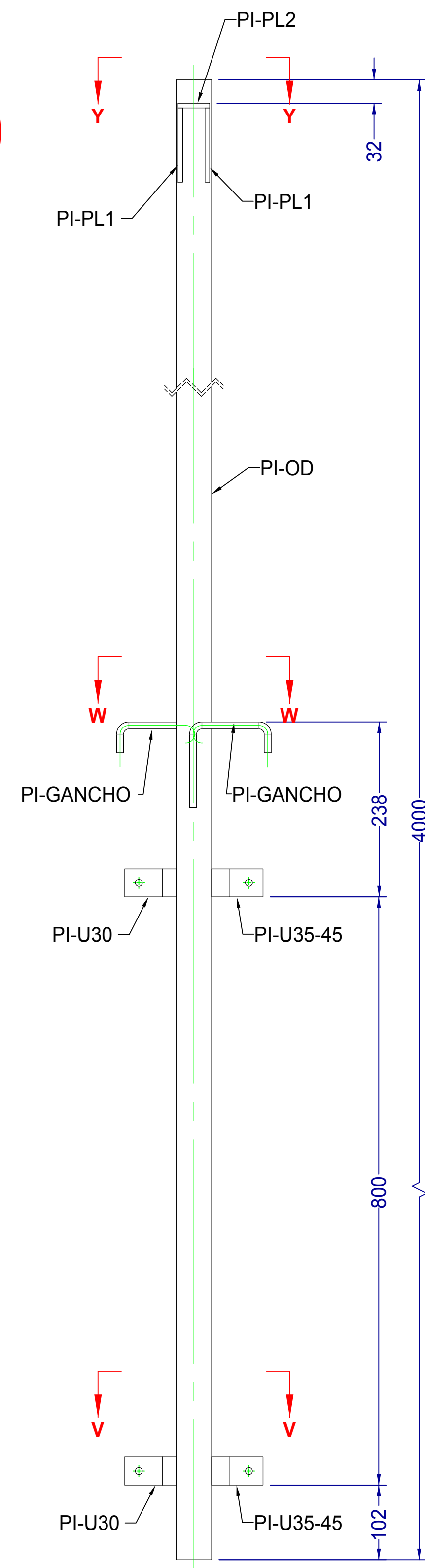
VISTA ELEVACIÓN PLUMA INSTALACIÓN
