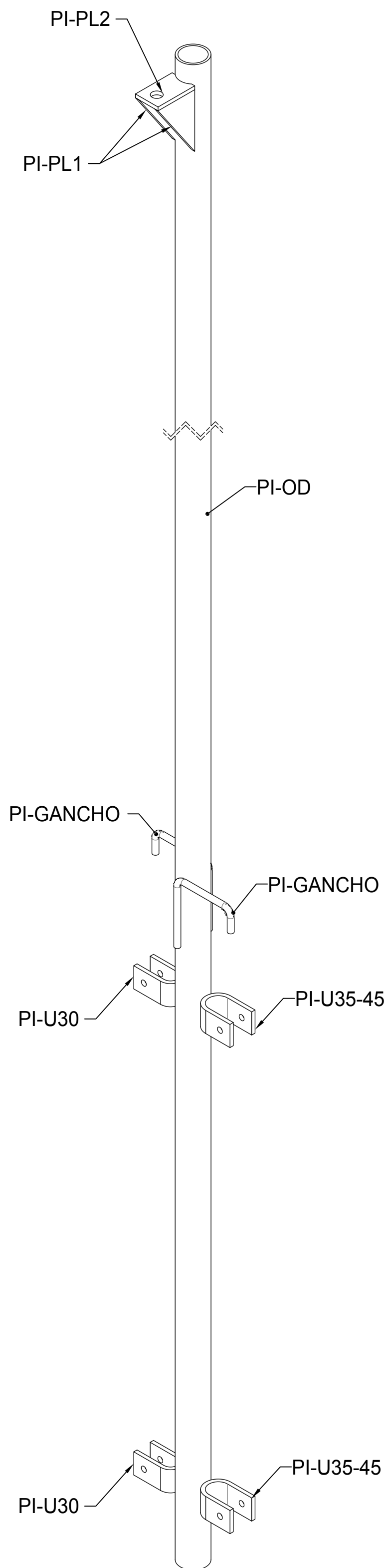
VISTA ISOMÉTRICA PLUMA INSTALACIÓN
